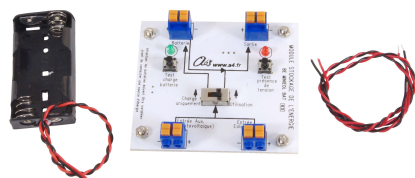
Module Chargeur* Réf. : BE-MINIEOL-BAT
