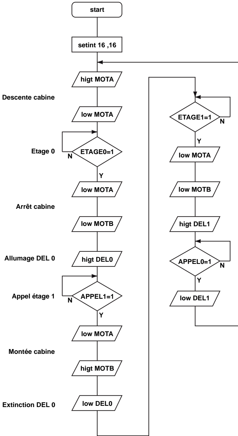
Programme EX5-Arrêt urgence.cad
