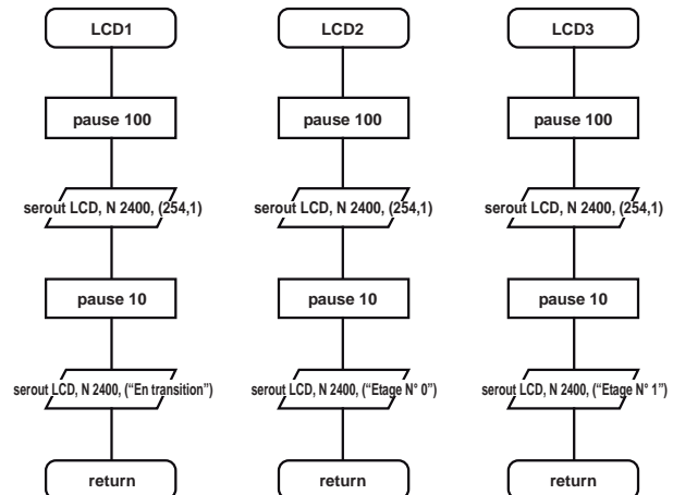
Sous programmes de gestion de l'afficheur
