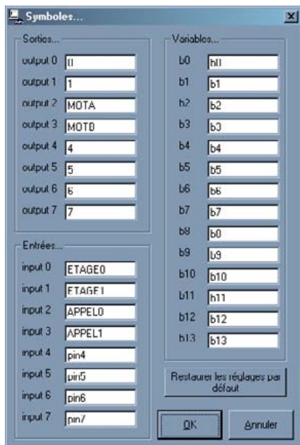
La table des symboles ci-dessus donne la correspondance entre les noms utilisés dans le programme et le numéro des entrées / sorties du boîtier de commande "AutoProg".
