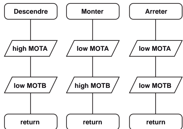
Sous programmes de gestion du déplacement de la cabine
