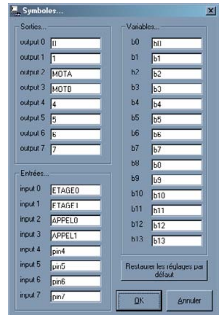
La table des symboles ci-dessus donne la correspondance entre les noms utilisés dans le programme et le numéro des entrées / sorties du boîtier de commande "AutoProg".
