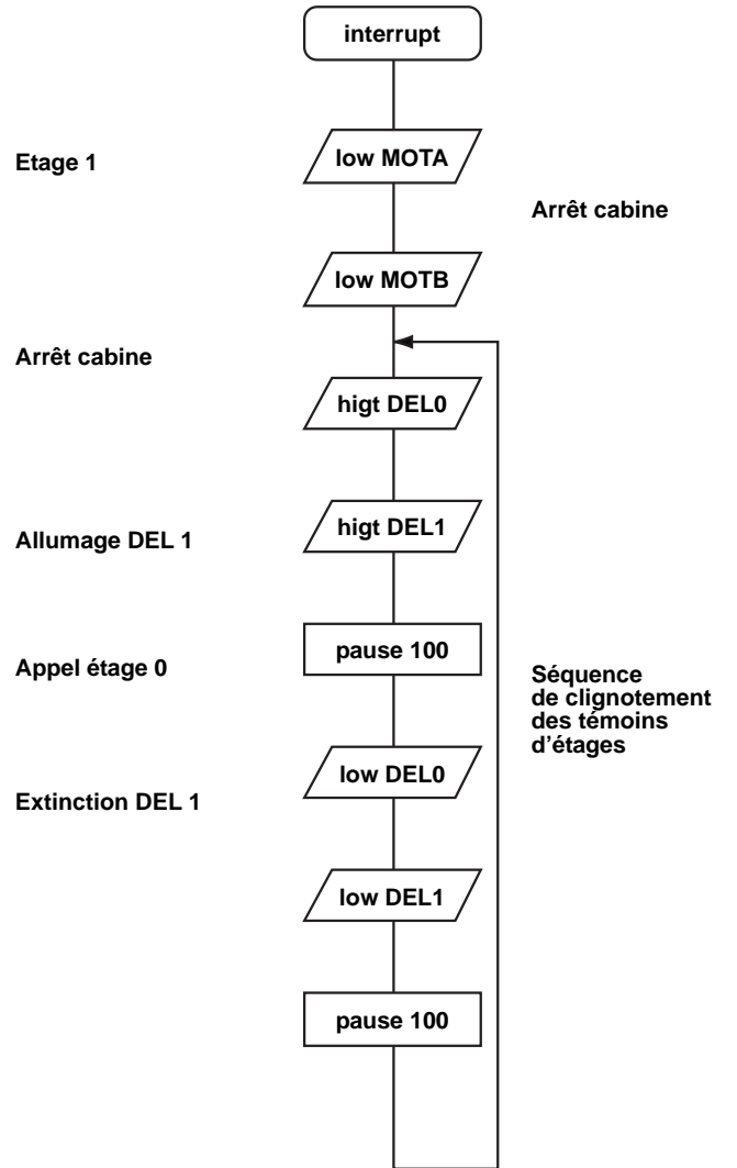
Sous programme de gestion d'interruption par bouton d'arrêt d'urgence
